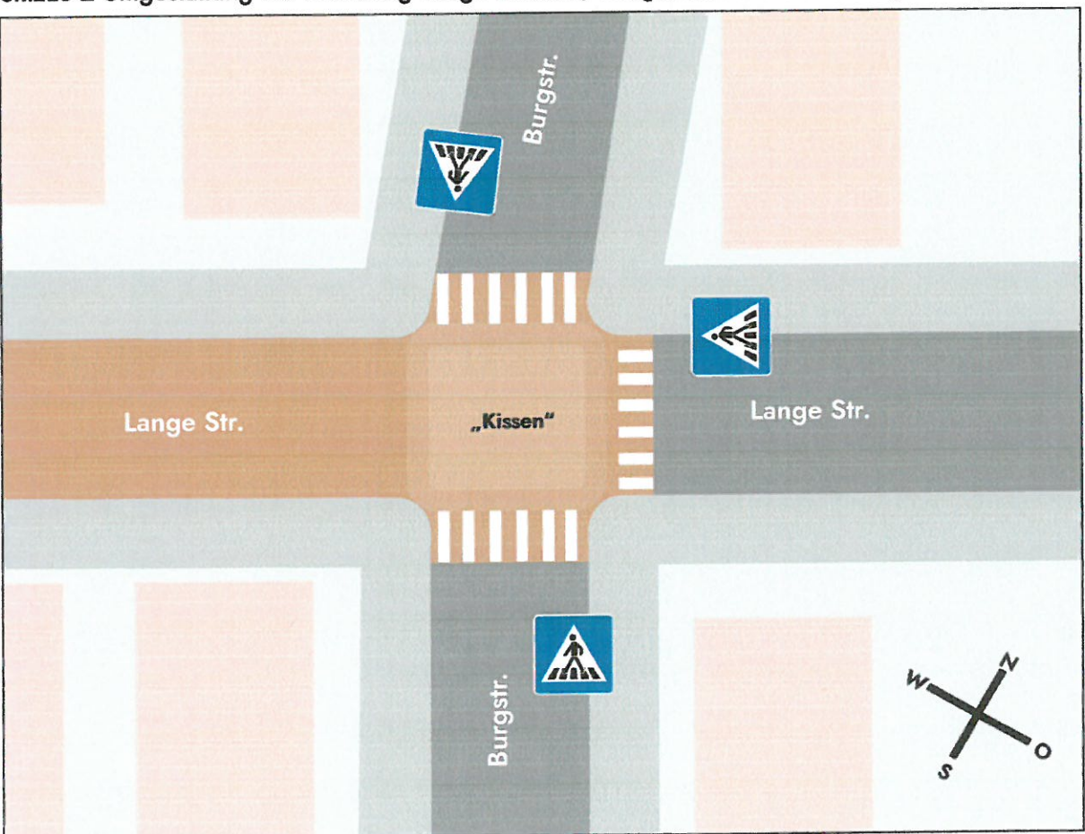
Skizze 2 Umgestaltung der Kreuzung Lange Strasse / Burgstrasse mit 3 Querungshilfen/Zebrastrreifen
