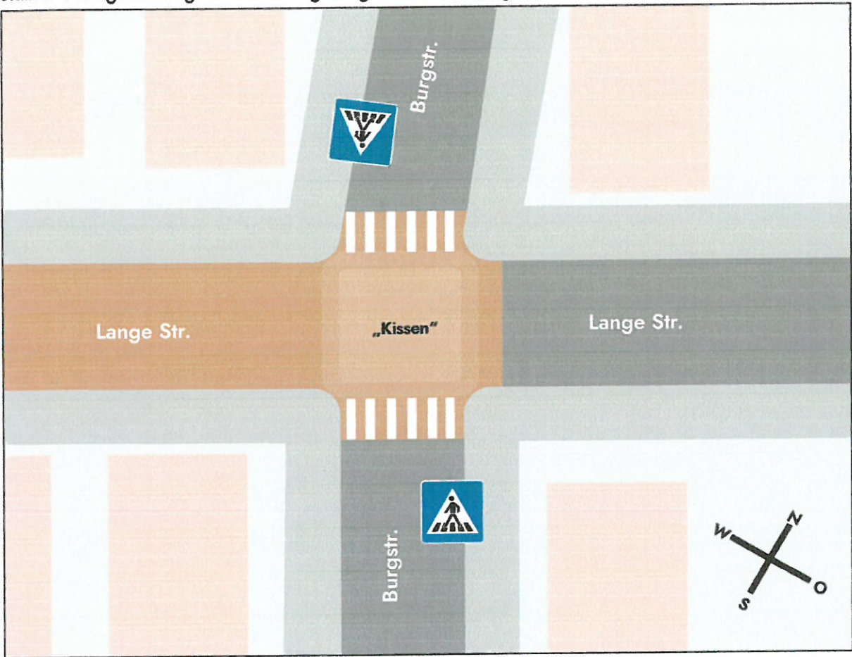
Skizze 1 Umgestaltung der Kreuzung Lange Strasse / Burgstrasse mit 2 Querungshilfen/Zebrastrreifen
